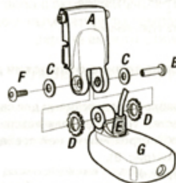
Рис. 4. Сборка датчика Piranha 1x-4x
