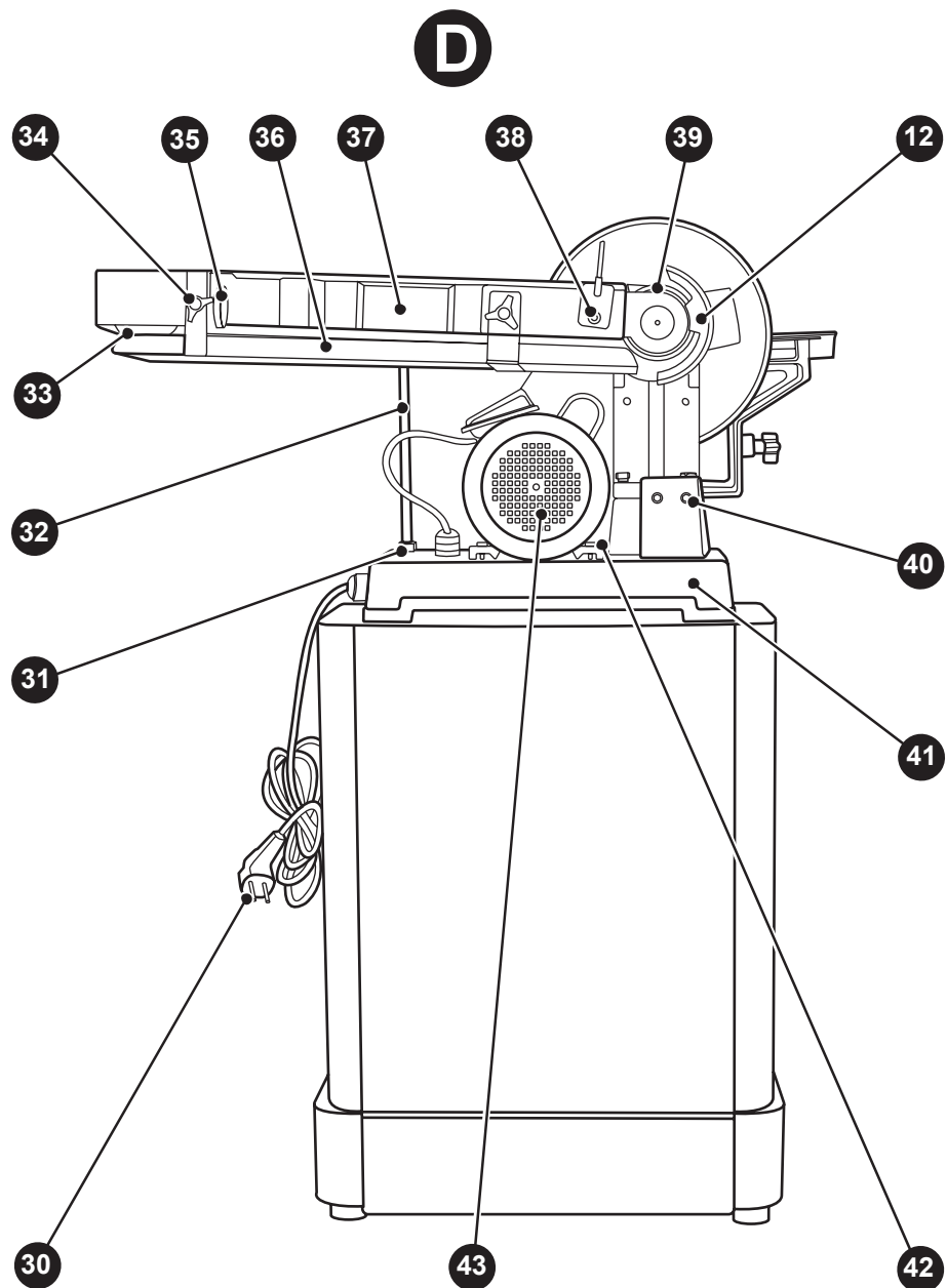
Рисунок D — общий вид станка.
