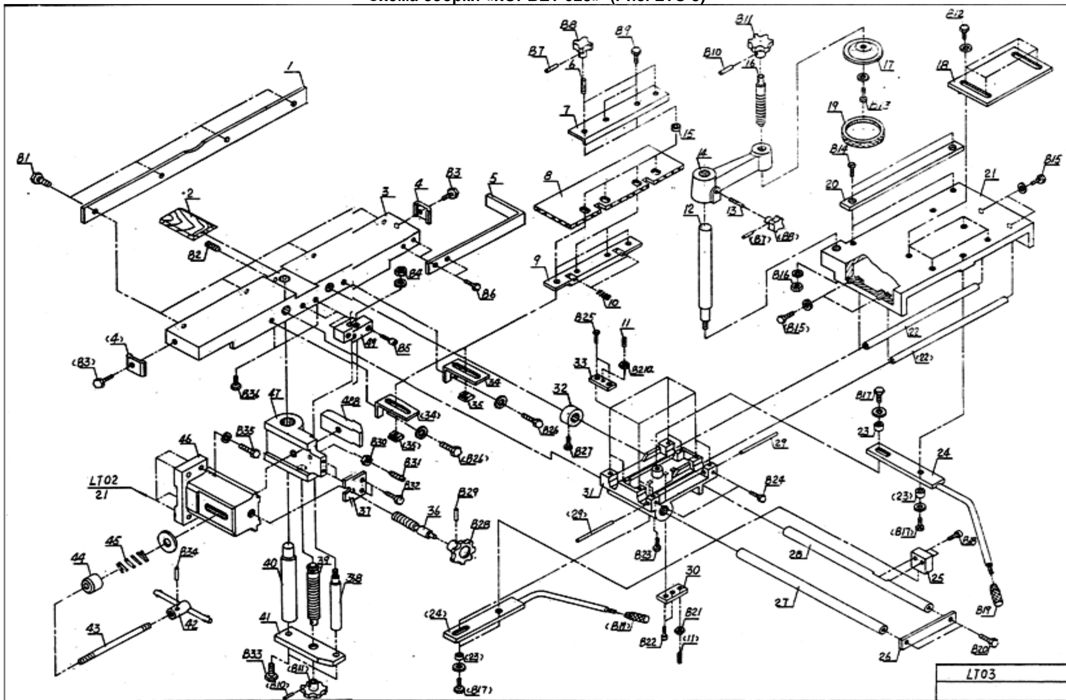
Схема сборки «КОРВЕТ 323» (Рис. ЛТО 3)
