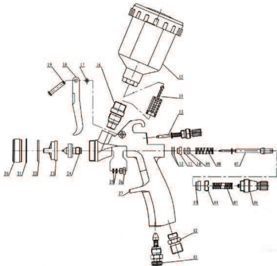
Рис. 5. Схема краскопульты модели КРП - 0,8/0,12 ВБ ПРОФИ:
