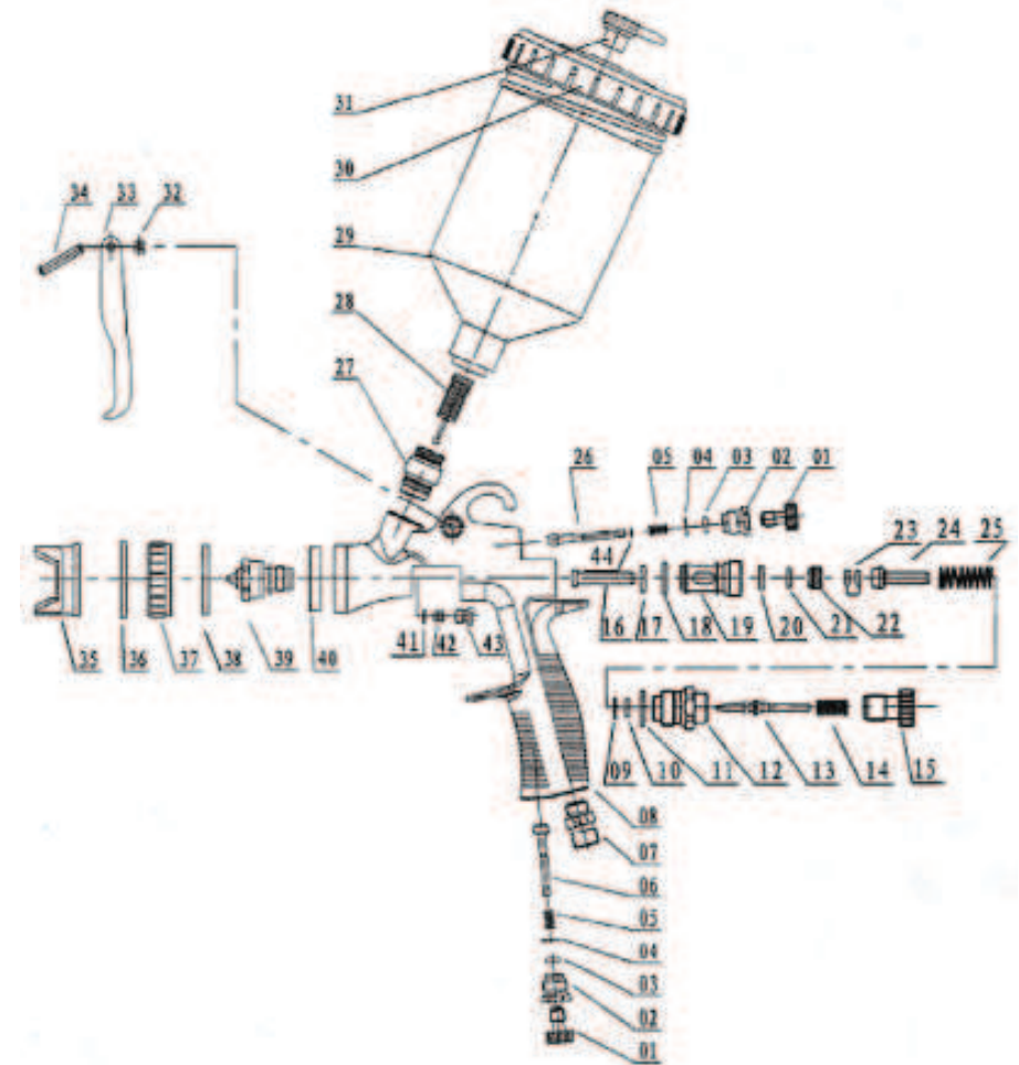
Рис. 4. Схема краскопульты модели КРП - 1,5/0,6 ВВ ПРОФИ:
