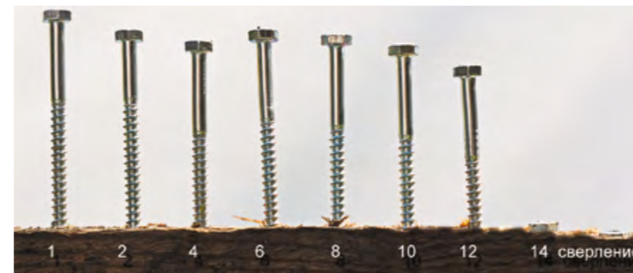
▲ Муфта регулировки момента мягкая. Первые ступени создают совсем незначительное усилие затяжки, а самые последние оптимальны для закручивания «глухаря» 6x90 мм в массив сосны.
