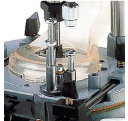
Быстрая установка глубины фрезерования 3-х позиционным револьверным упором.
