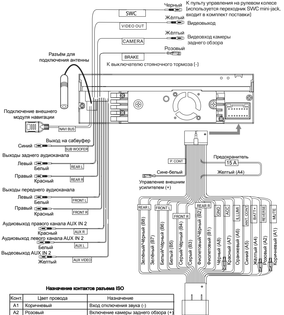
Разъём ISO
