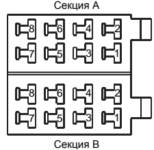
Расположение контактов разъема ISO:
